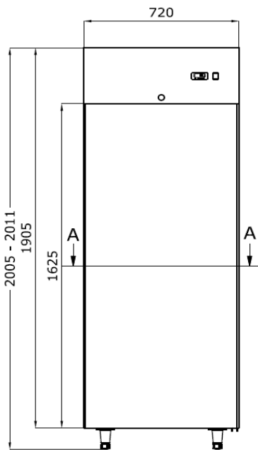
SN-711SG A-A
