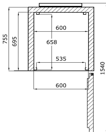
SN-711SG A-A
